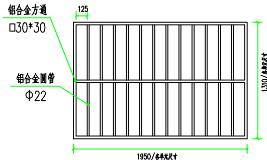
铝合金防盗网大样图
