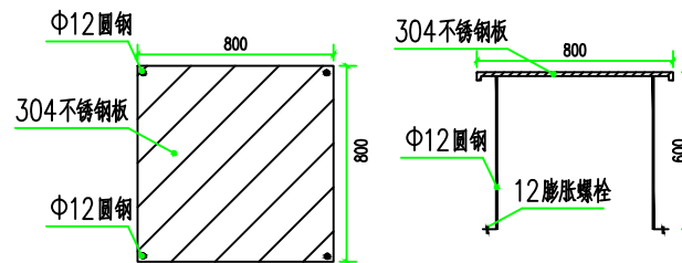
304不锈钢防雨烟罩
